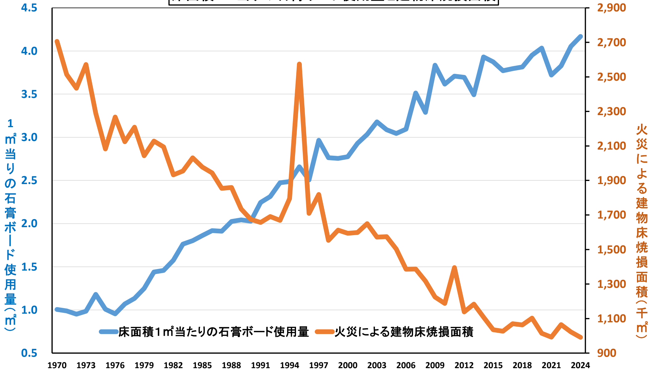
床面積1㎡当りの石膏ボード使用量と建物床焼損面積
